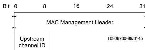
Figure C.6-32/J.112 – UCC-RSP message
