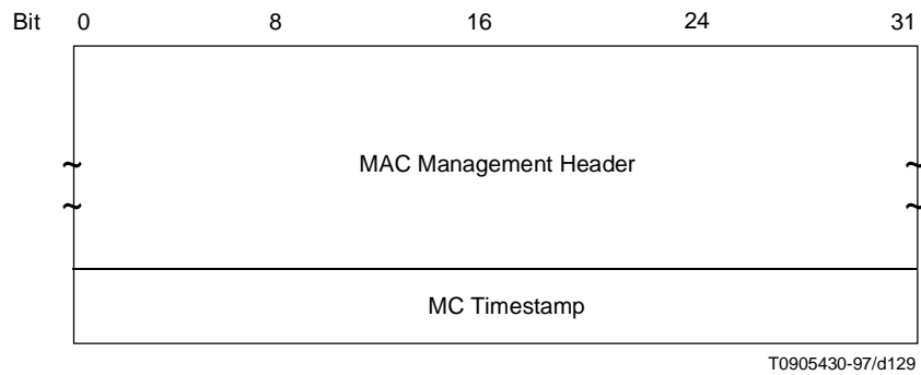
Figure C.6-16/J.112 – SYNC Message
