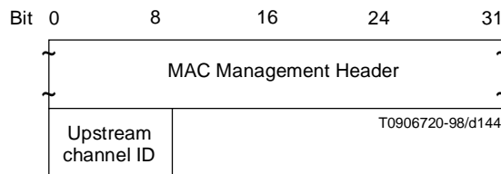
Figure C.6-31/J.112 – UCC-REQ message
