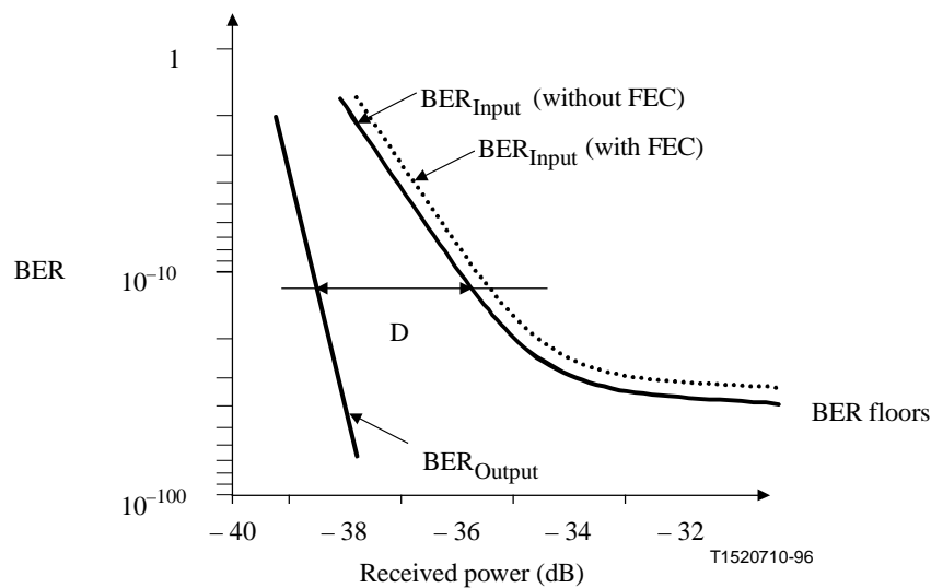
Figure 7/G.975 – Coding gain (D) evaluation scheme
